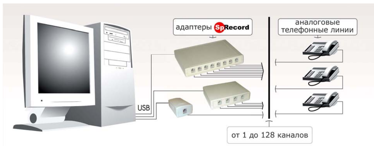
Рисунок 1. Система SpRecord
